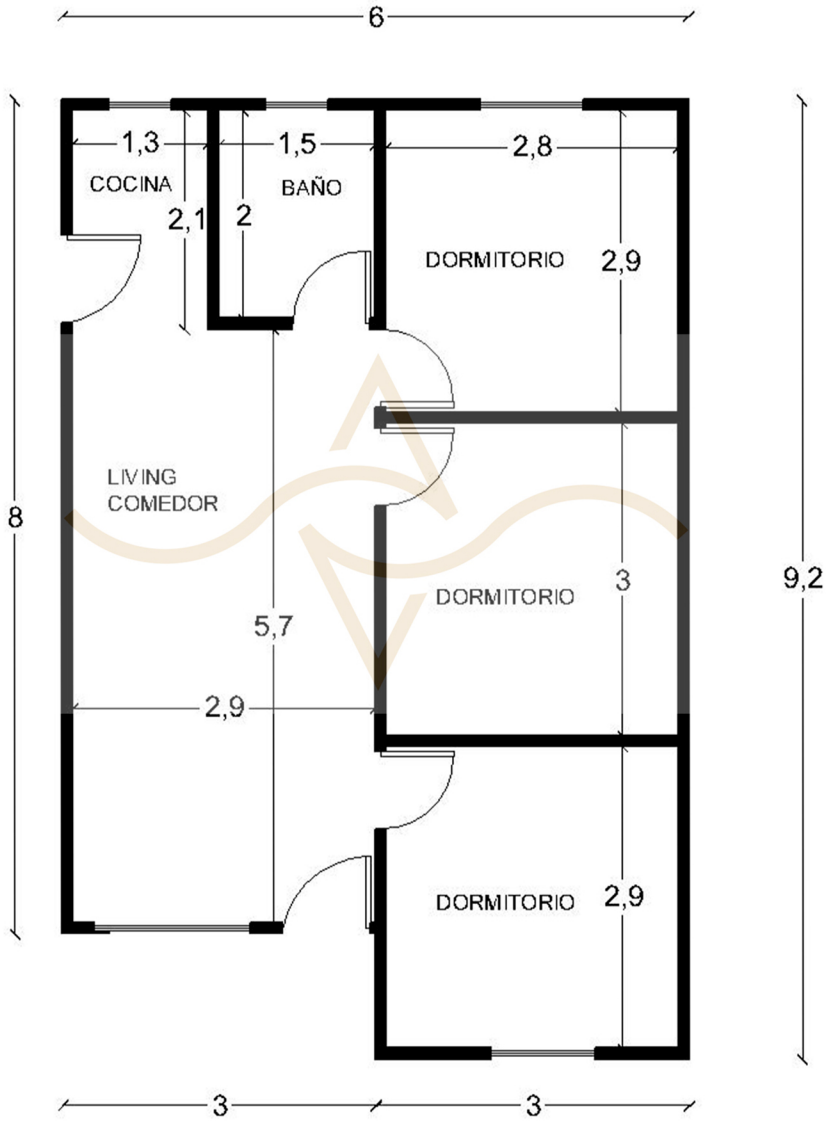
Plano Planta
